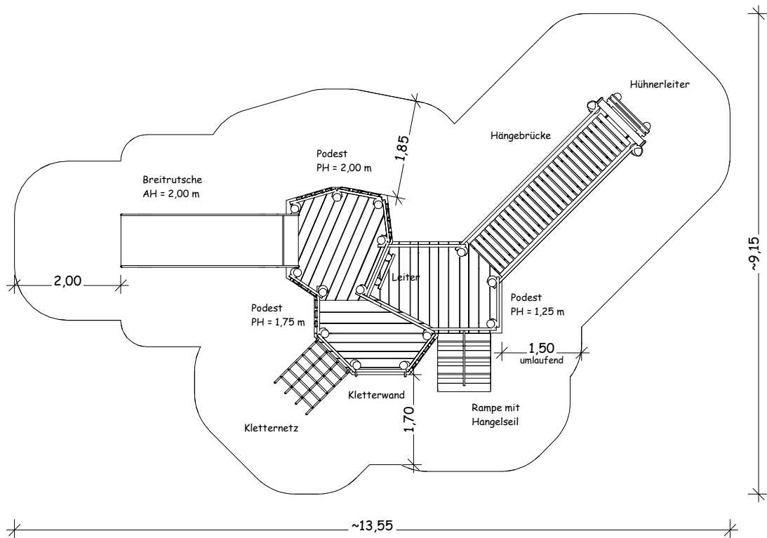
Draufsicht
