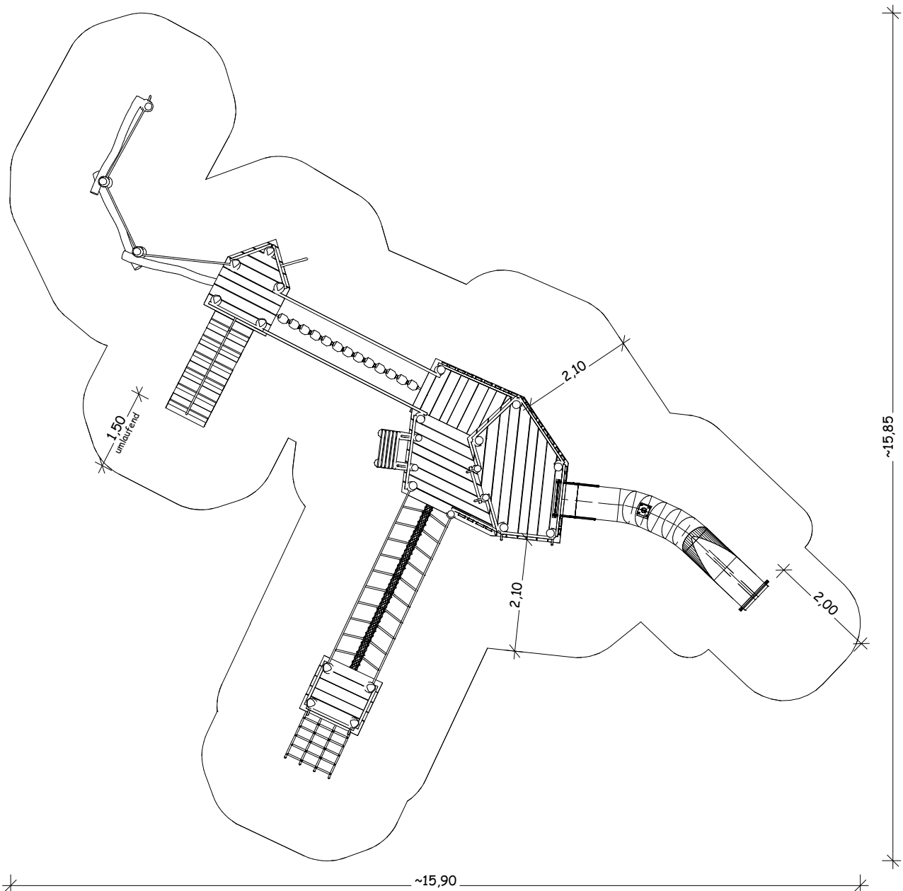
Draufsicht
