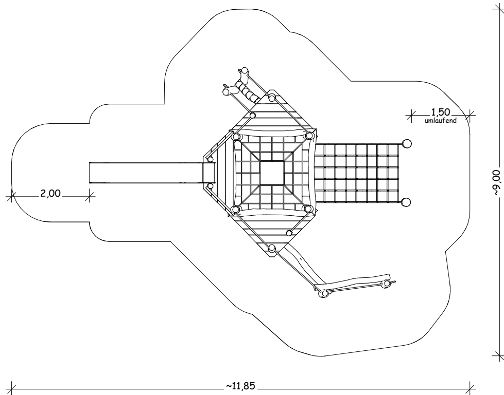
Draufsicht
