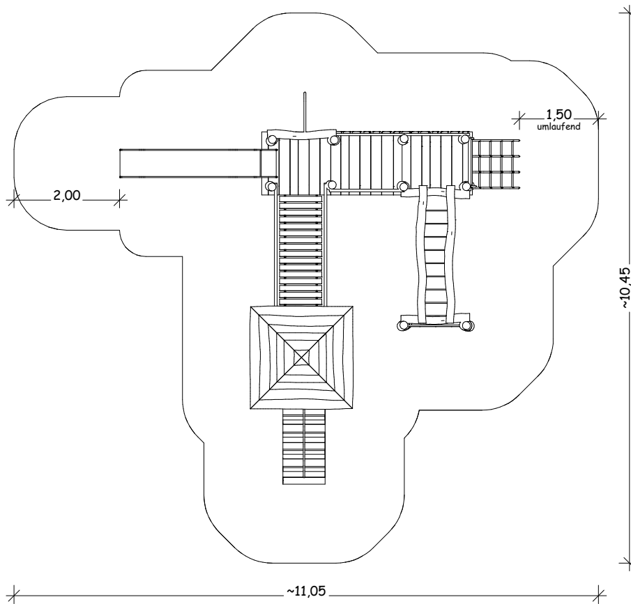
Draufsicht
