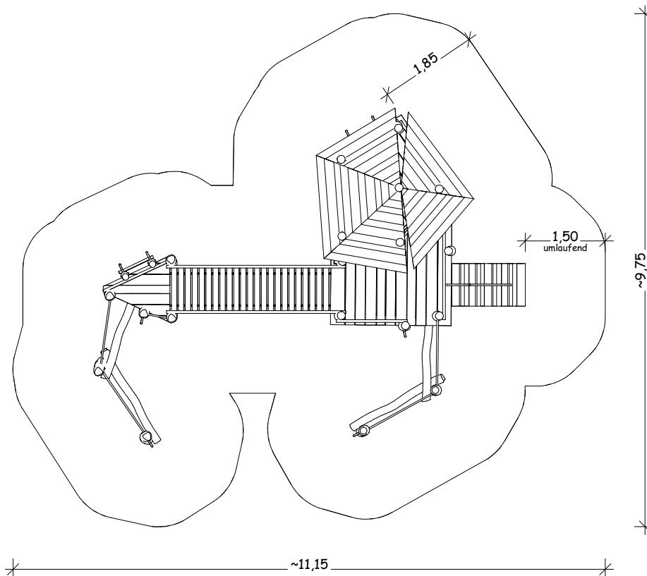
Draufsicht
