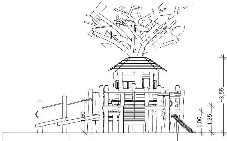
Ansicht (mit Baum)
