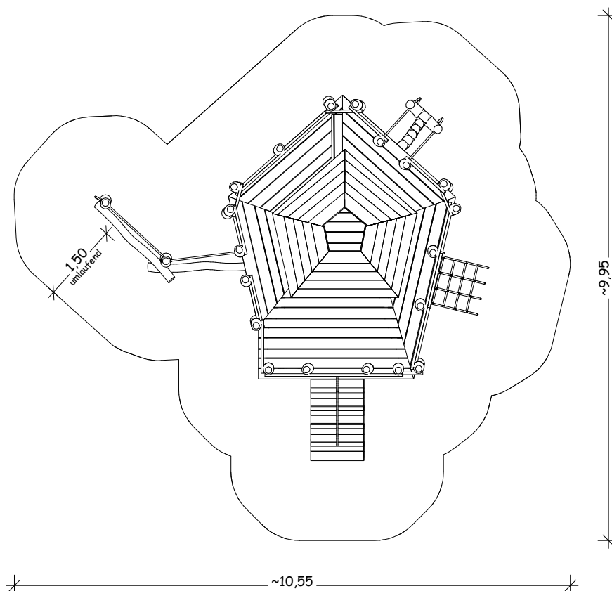
Draufsicht (ohne Baum)
