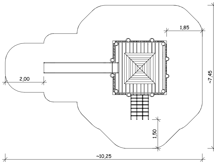
Draufsicht
