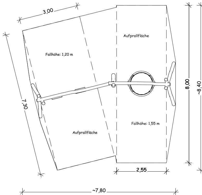
Draufsicht
