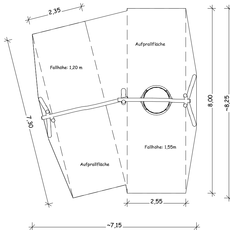
Draufsicht
