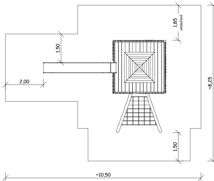
Draufsicht
